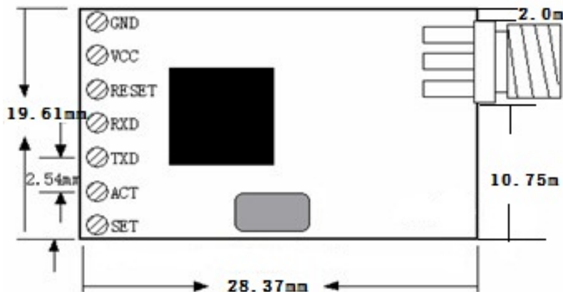
BM100N 尺寸示意图
