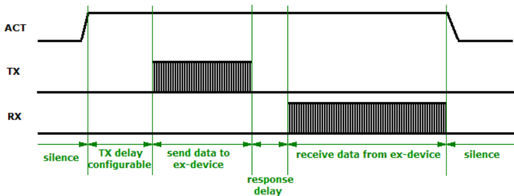
外设响应的 ACT、TX 和 RX 时序图
