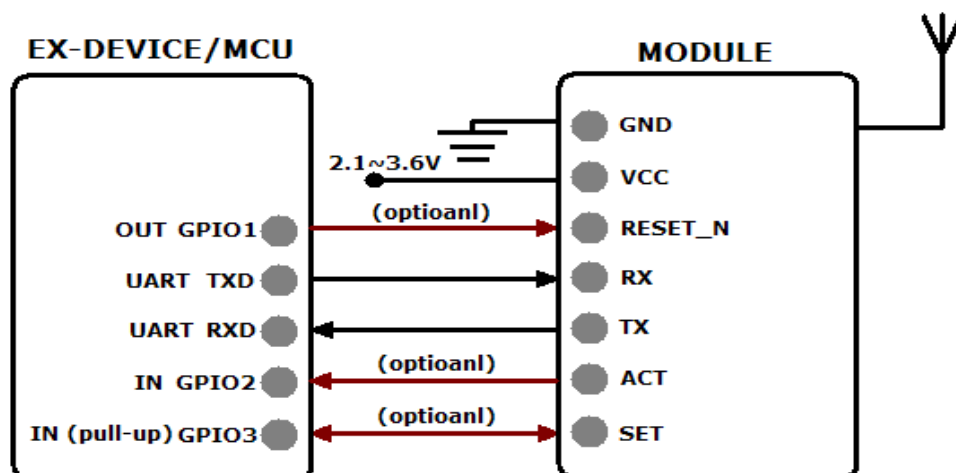
BM100N 与外设的连接示意图
